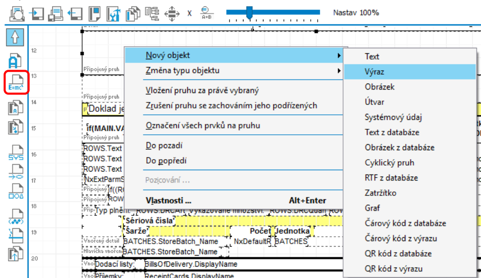
Obr. 08 – Vložení výrazu
